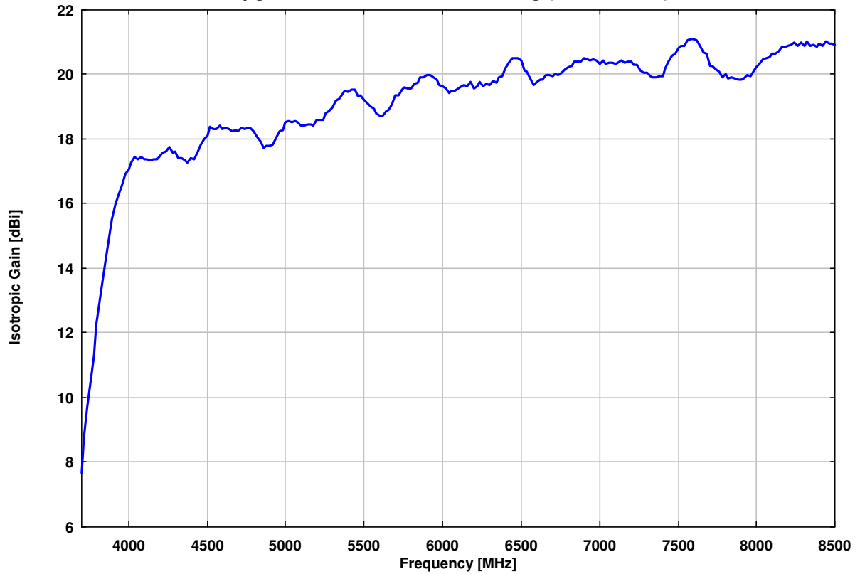
Isotropgewinn bei 1 m Messentfernung (Vorderkante)
